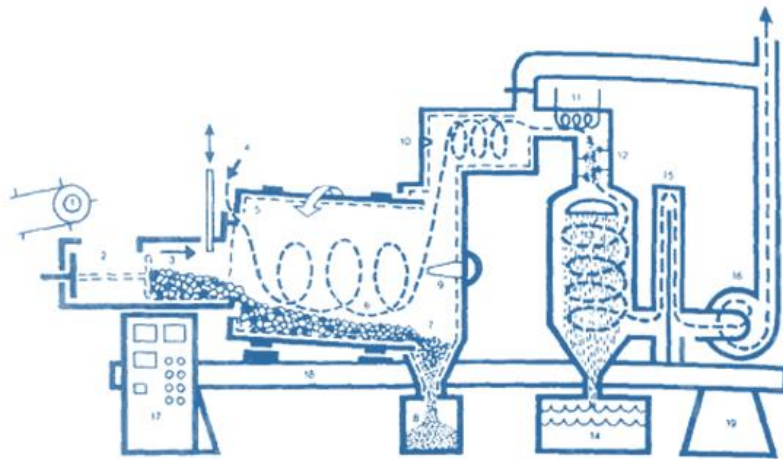
ภาพเตาเผาแบบหมุน
