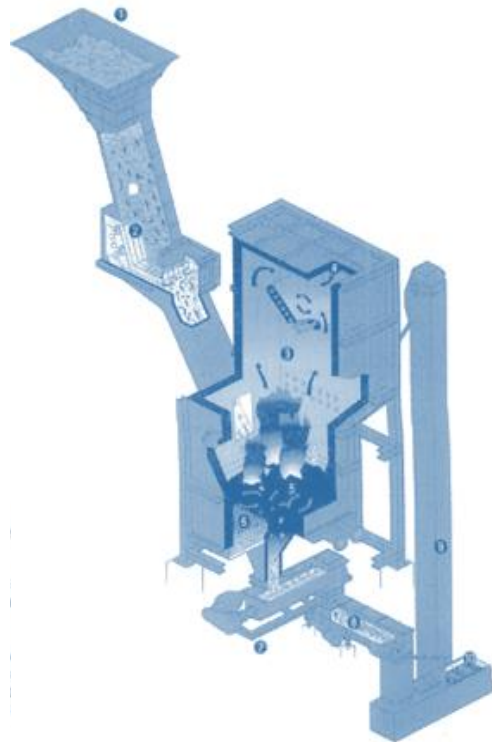
ภาพเตาเผาแบบฟลูอิดไดซ์เบด
